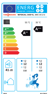
Etykieta klasy efektywności energetycznej (ErP) pompy ciepła Vitocal 300-G, BWC 301.C12
